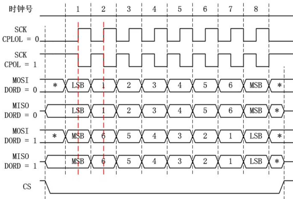
图 16-1: SPI 通讯时序 (CPHA = 0)
