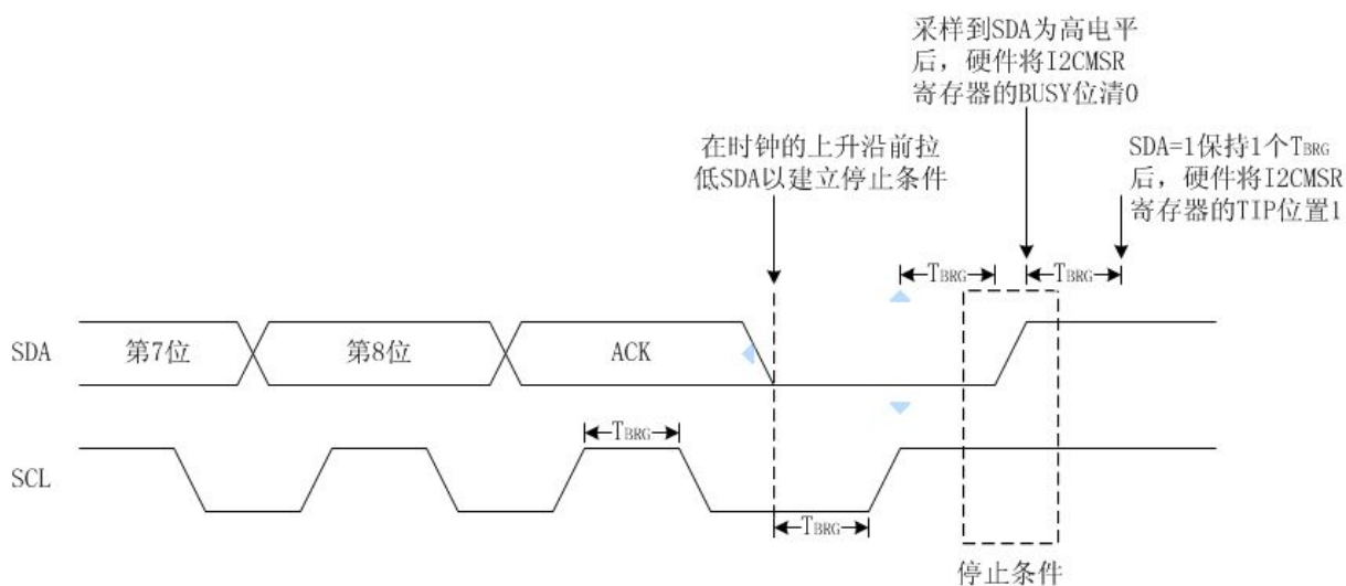
图 17-7： 主控模式停止条件时序
