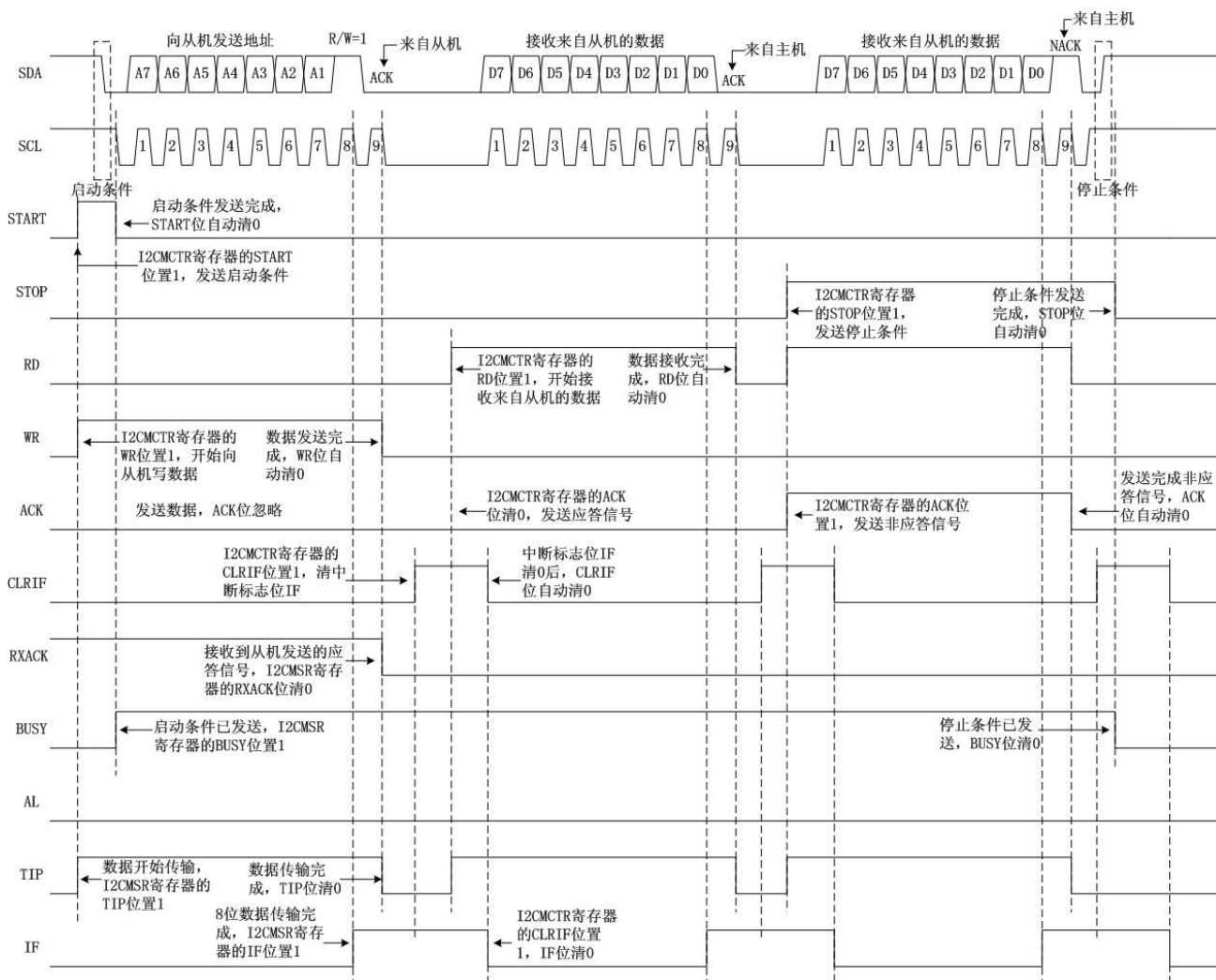
图 17-10： 主控模式接收时序图
