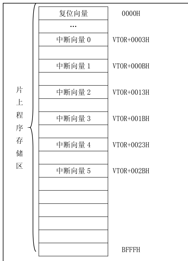
图 2-1: CBM63xx 的程序存储器映射
