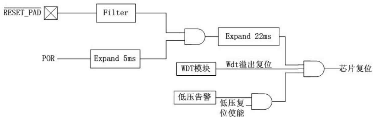
图 5-1： 片上复位电路的简化框图
