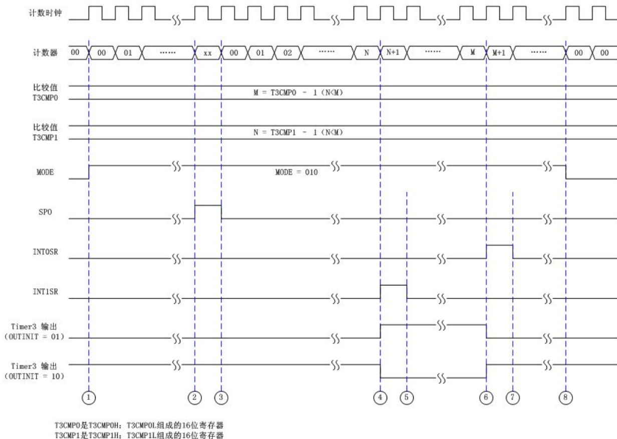
图 11-4: Timer3 单脉冲输出工作时序图
