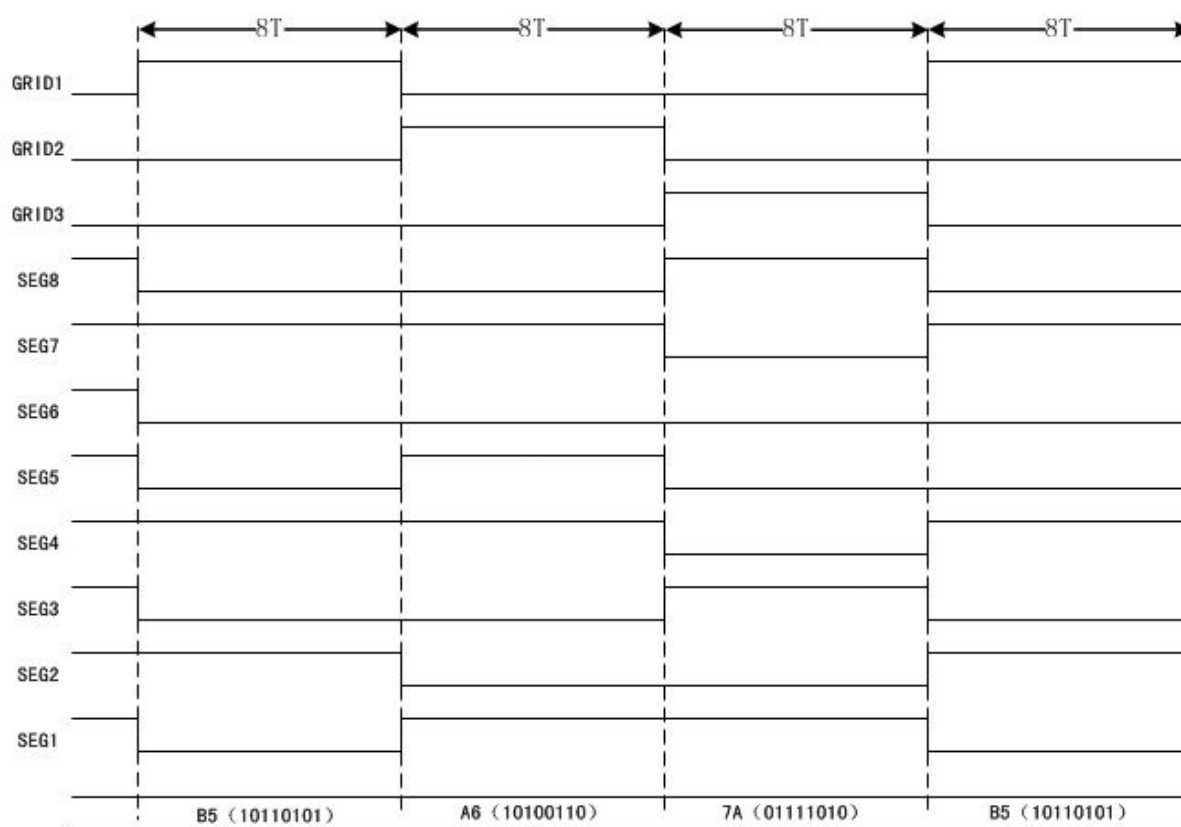
图 19-1: LED 显示控制时序图(共阳极)
