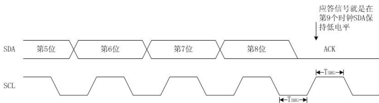
图 17-8： 主控模式应答时序图
