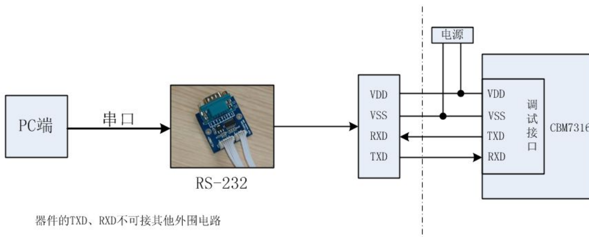
图 5-7： 典型的在线调试连接方式
