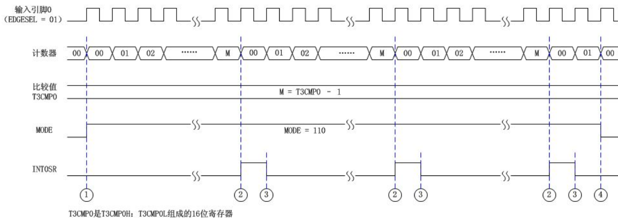
图 11-3: Timer3 外部事件计数工作时序图
