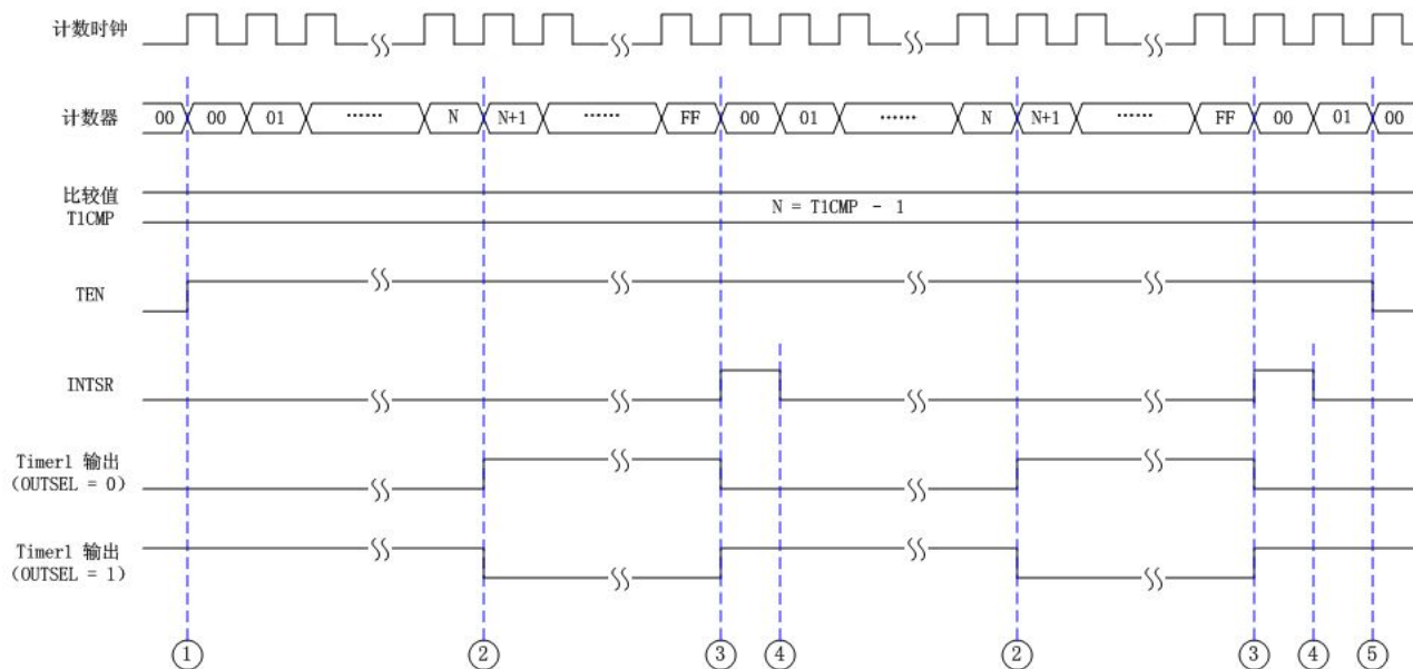
图 9-2: Timer1 PWM 输出工作时序图 (T1CMP \neq 0)
