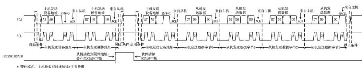
图 17-2: 硬件标准模式主机读时序图(只读)
