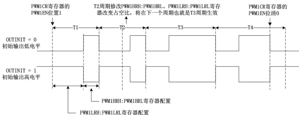
图 12-1： PWM1 输出的工作原理
