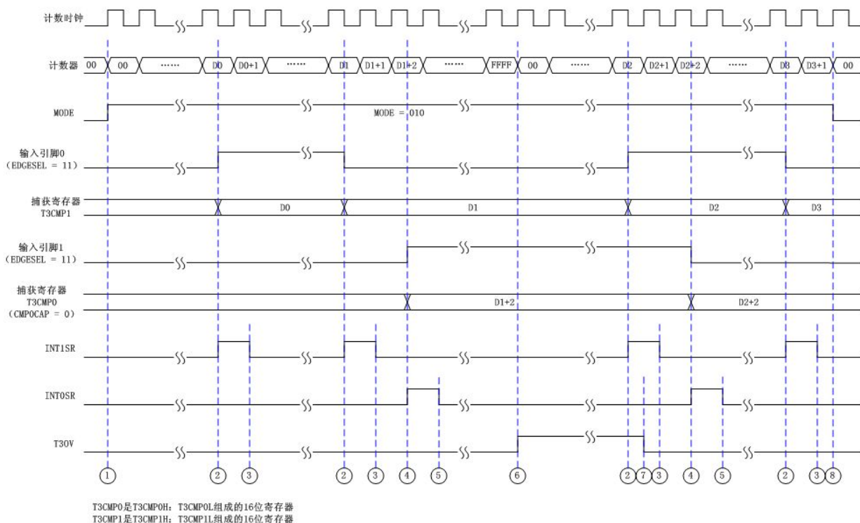
图 11-6: Timer3 使用两组捕获寄存器测量两个输入电平的宽度工作时序图
