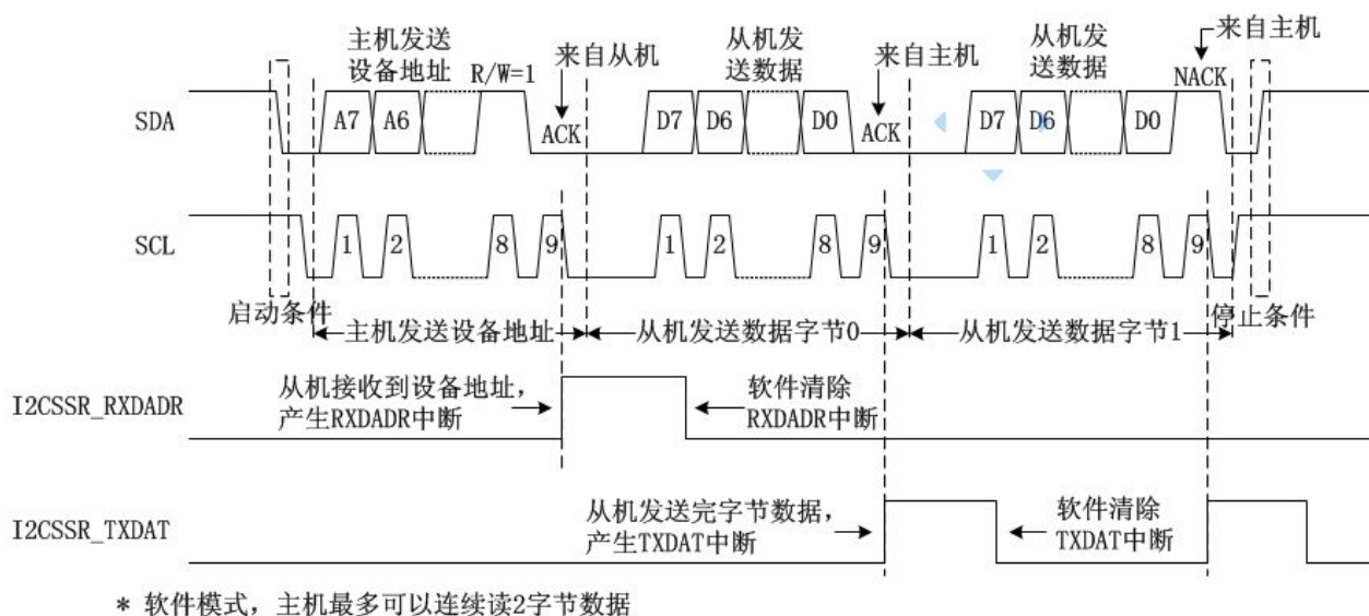
图 17-3：软件快速模式主机读时序图(只读)
