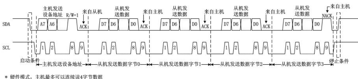
图 17-1: 硬件快速模式主机读时序图(只读)
