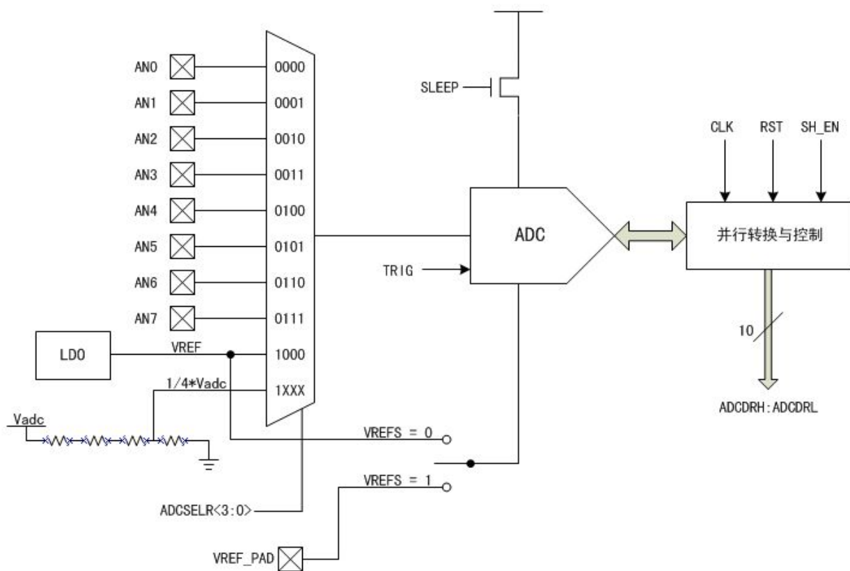
图 13-1: ADC 的框图
