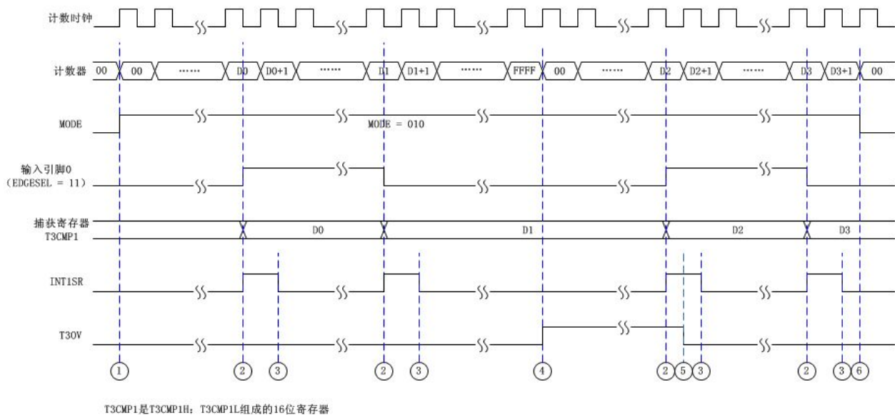
图 11-5: Timer3 使用一组捕获寄存器测量一个输入电平的宽度工作时序图
