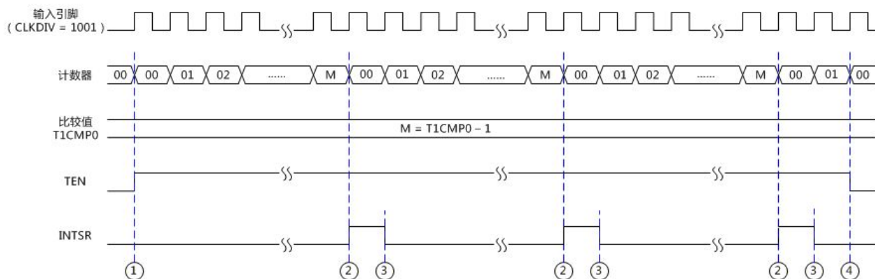
图 9-3: Timer1 外部事件计数工作时序图
