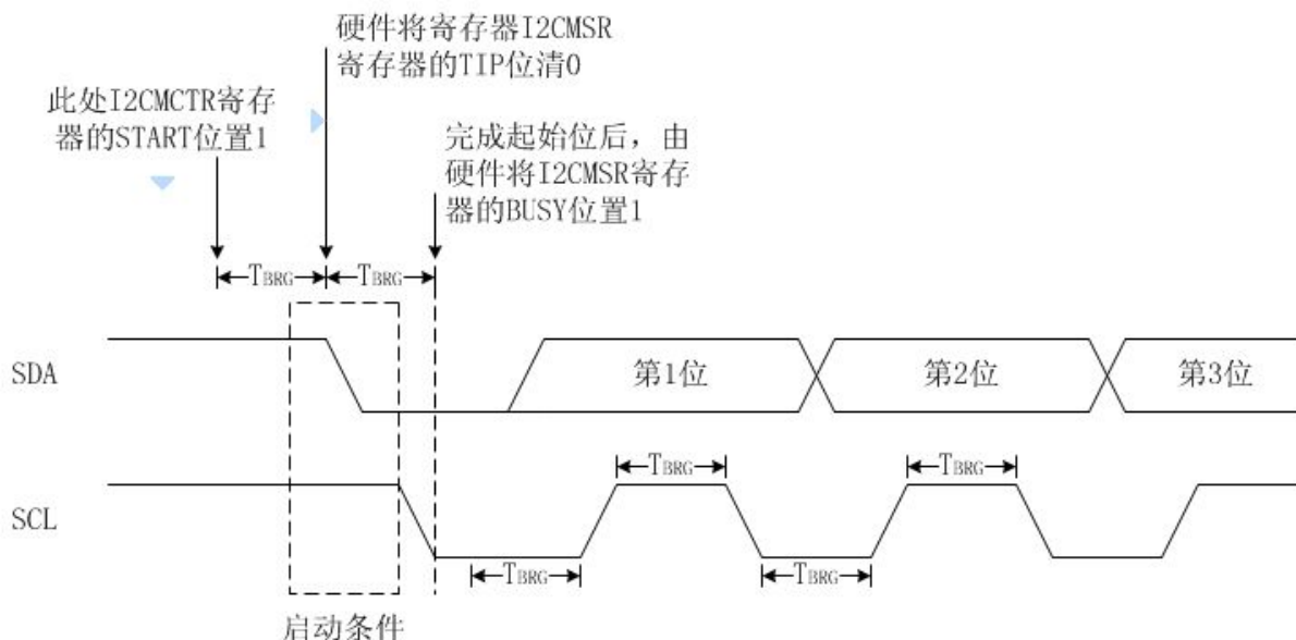
图 17-6： 主控模式启动条件时序
