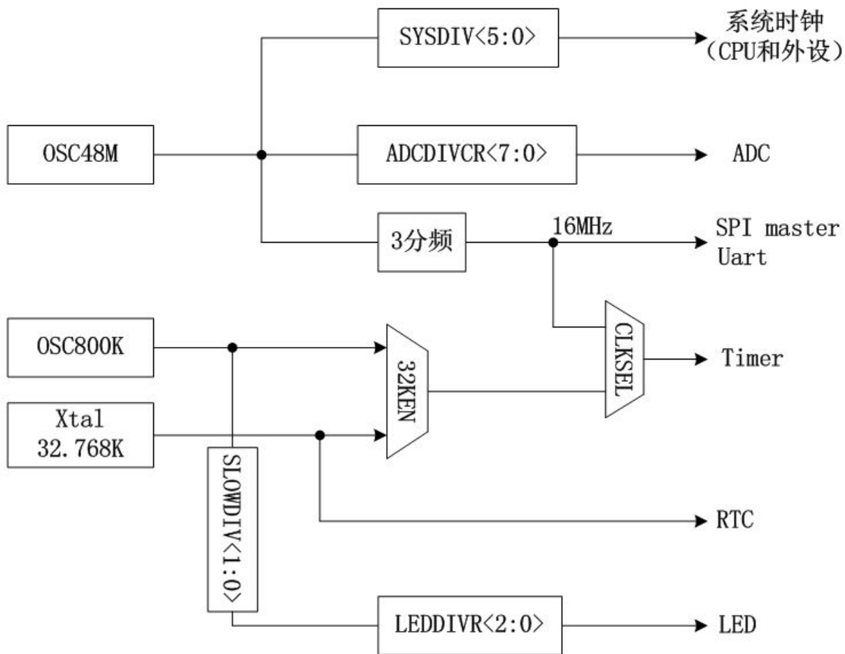
图 4-1: MCU 时钟源简化框图
