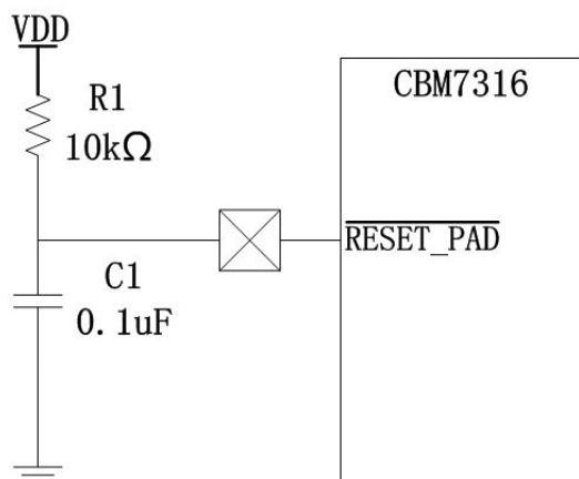
图 5-2: 推荐的外部复位电路
