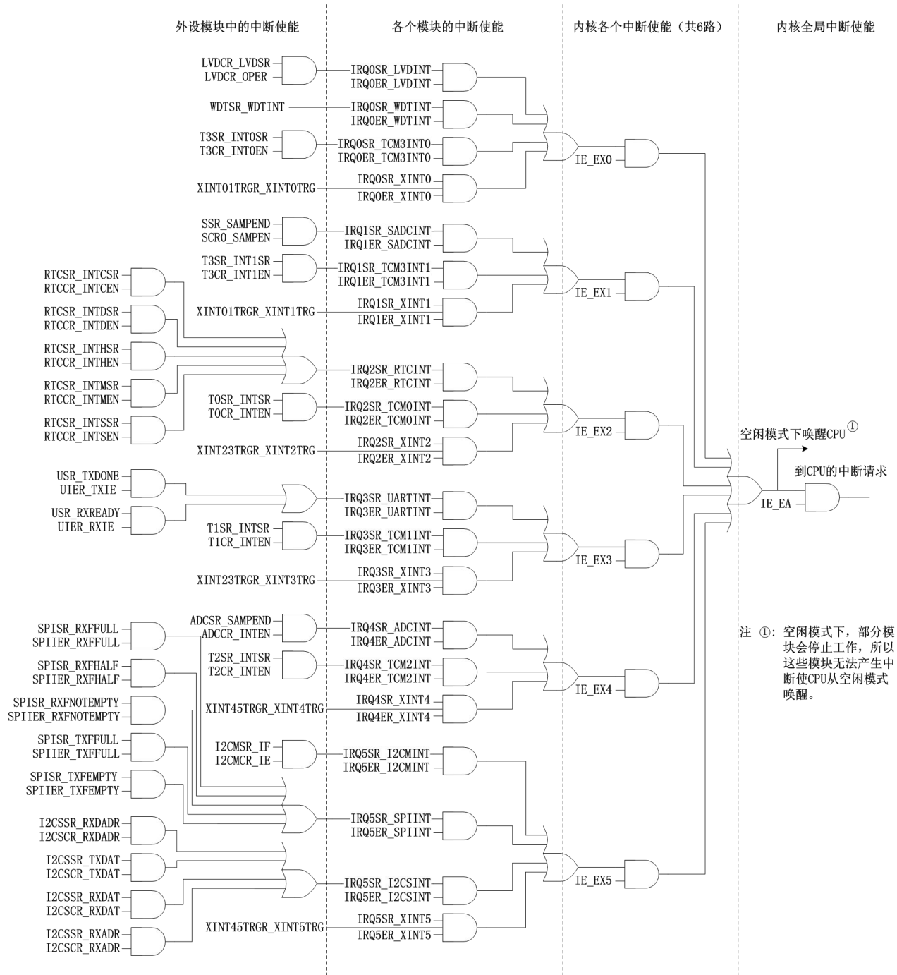
图 5-4：中断控制逻辑图
