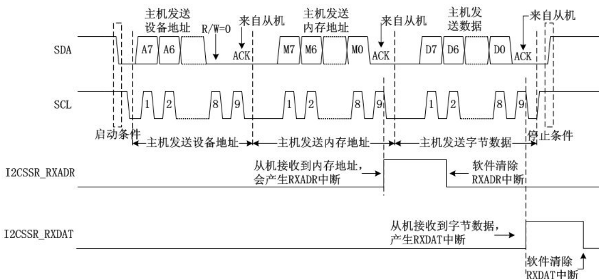
图 17-4： 软件标准模式主机写时序图
