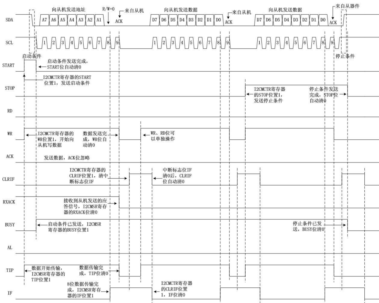
图 17-9： 主控模式发送时序图
