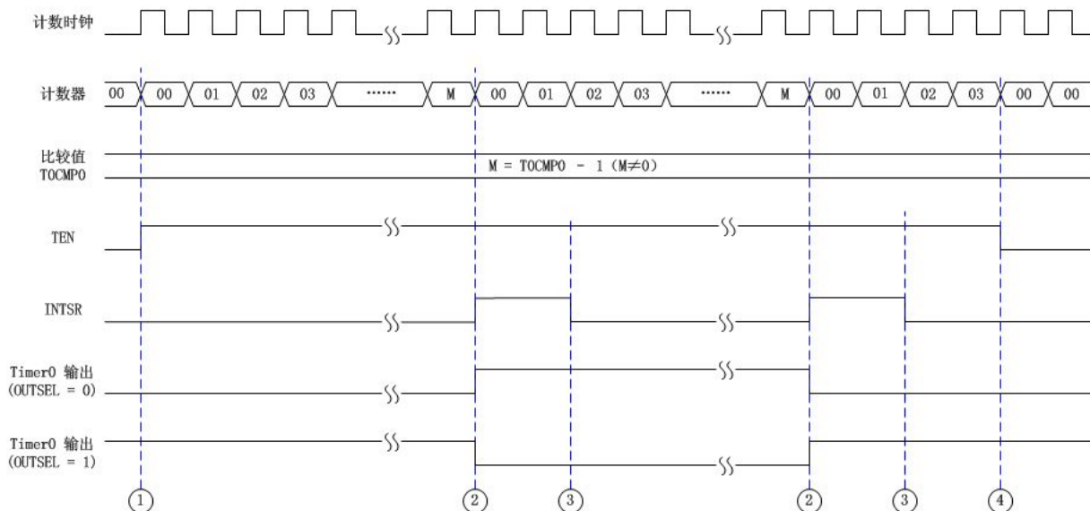
图 8-1: Timer0 间隔定时/方波输出工作时序图 (TOCMP0 ≠ 1)
