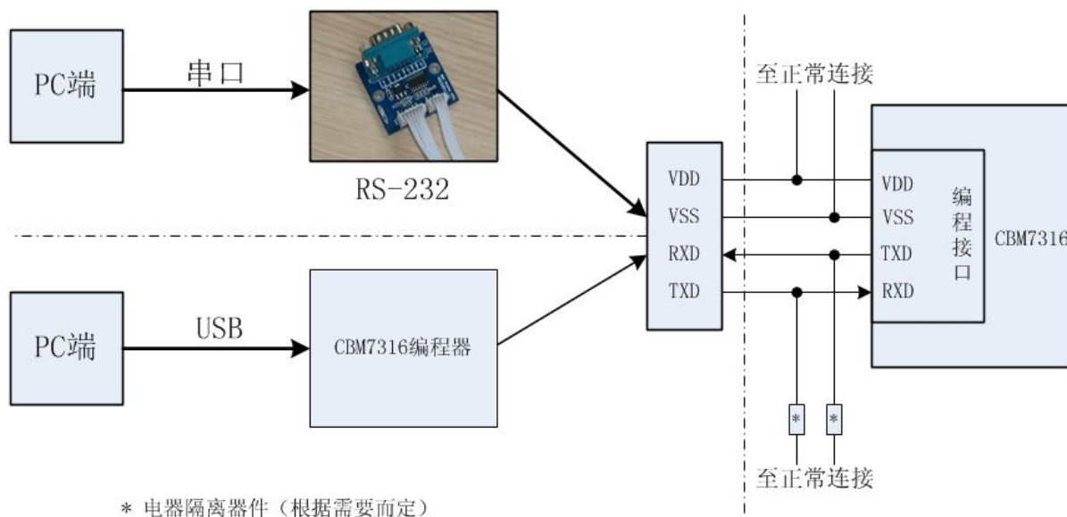
图 5-6: 典型的在线串行编程连接方式
