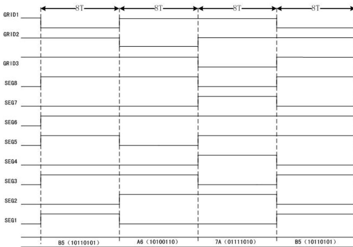
图 19-2: LED 显示控制时序图(共阴极)
