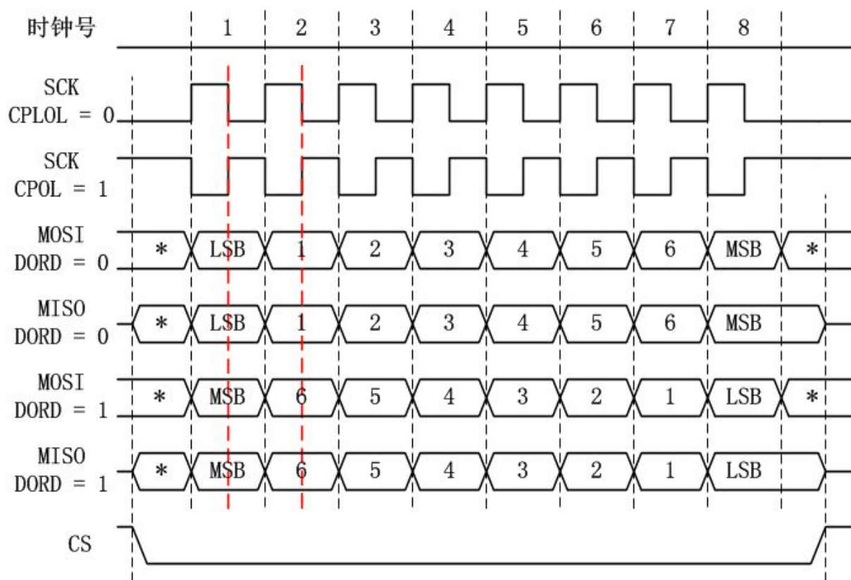
图 16-2: SPI 通讯时序 (CPHA = 1)
