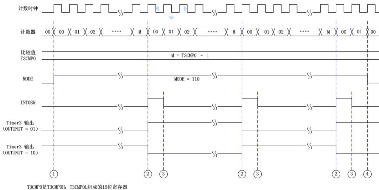
图 11-1: Timer3 间隔定时/方波输出工作时序图
