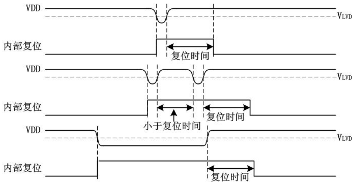
图 5-3: 低压复位情形
