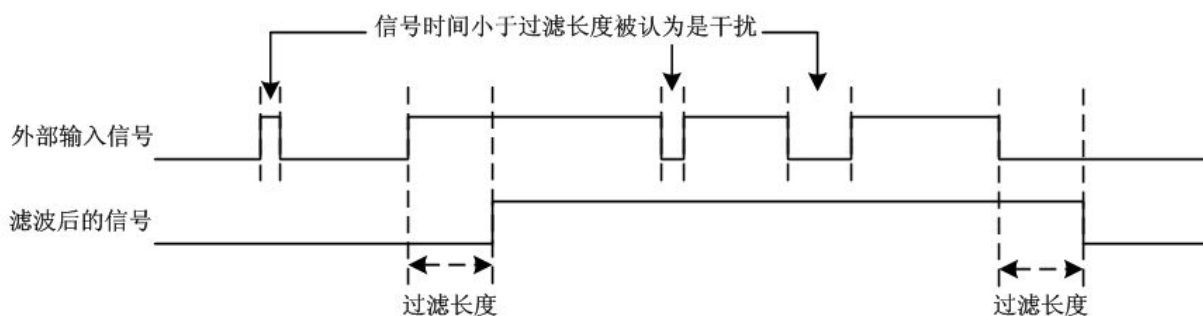
图 5-5： 外部中断信号滤波处理
