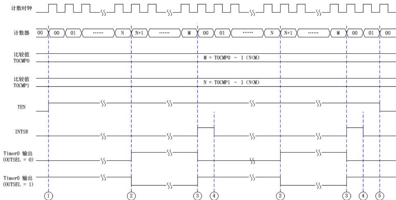
图 8-2: Timer0 PWM 输出工作时序图 (TOCMP0 \neq 1, TOCMP1 < TOCMP0)
