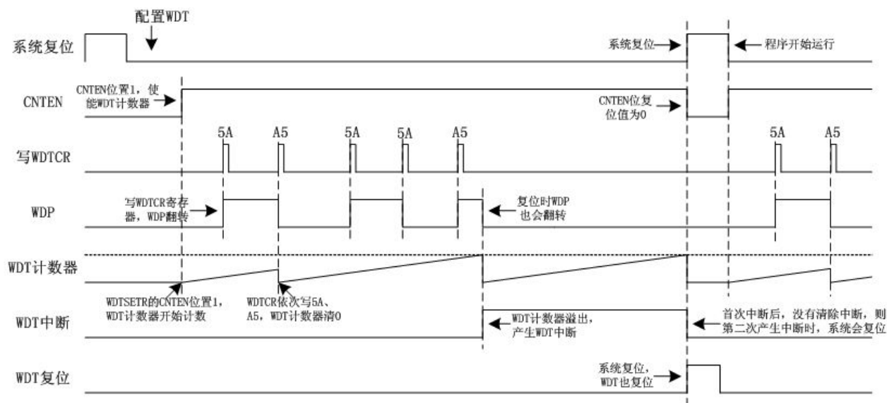
图 7-1: 看门狗定时器工作时序图
