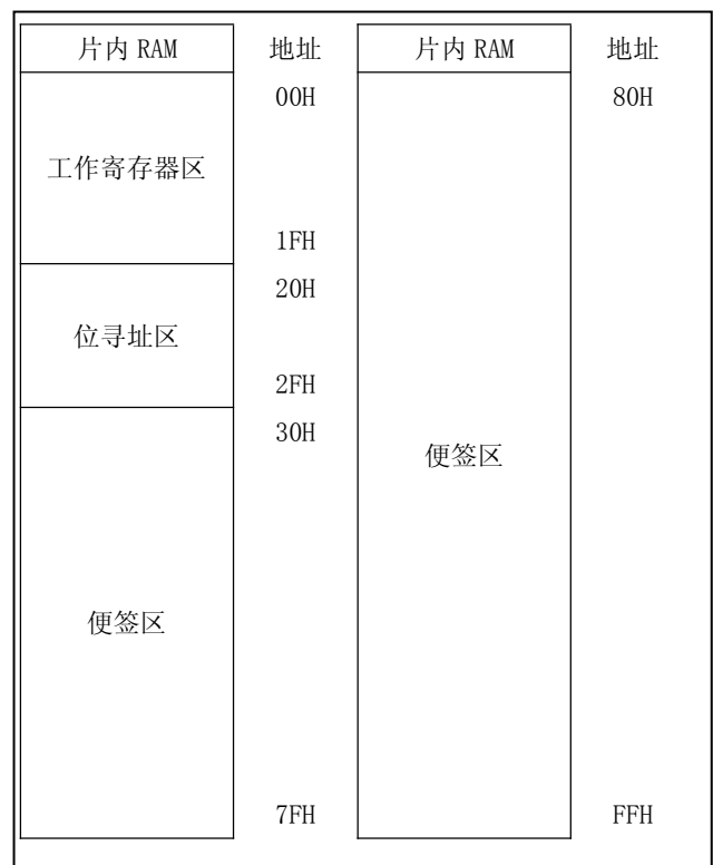
图 2-2: CBM63xx 片内 RAM 映射
